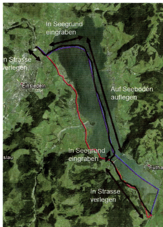
Mögliche Linienführungen der Abwasserleitung L1 zwischen der ARA Oberes Sihltal und der ARA Einsiedeln. Linienführung TBF + Partner AG: Variante rot = entlang Strasse. Variante blau = Seedruckleitung. Linienführung Holinger AG: Variante schwarz = Kombination Strasse und Seedruckleitung. Illustrationen: zvg
